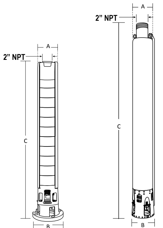
Acoplamiento NEMA 6"
